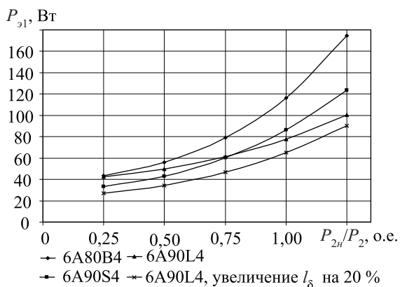
Рис. 3. Зависимость электрических потерь в статоре асинхронных двигателей от мощности (базовый 6А80В4, P_{2н}=0,75 кВт)
