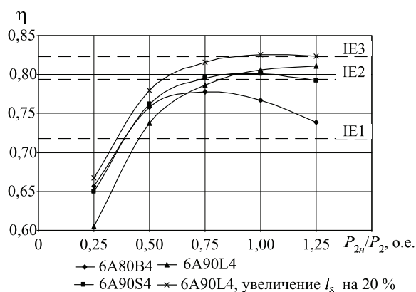
Рис. 2. Зависимость КПД асинхронных двигателей от мощности (базовый 6А80В4, P_{2н}=0,75 кВт)
