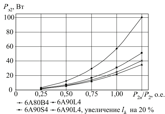
Рис. 4. Зависимость электрических потерь в роторе асинхронных двигателей от мощности (базовый 6А80В4, P_{2н}=0,75 кВт)
