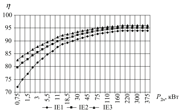
Рис. 1. Уровни КПД для нового стандарта энергоэффективности
